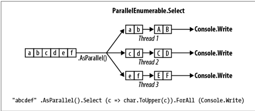
Figure 23-3. PLINQ ForAll
